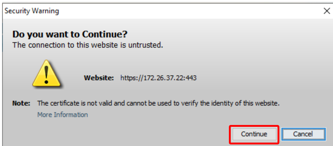
شکل ۳۲ - Security Warning
