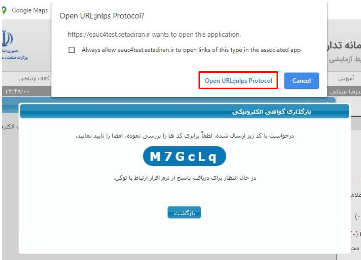
شکل ۳۰ - Open URL
